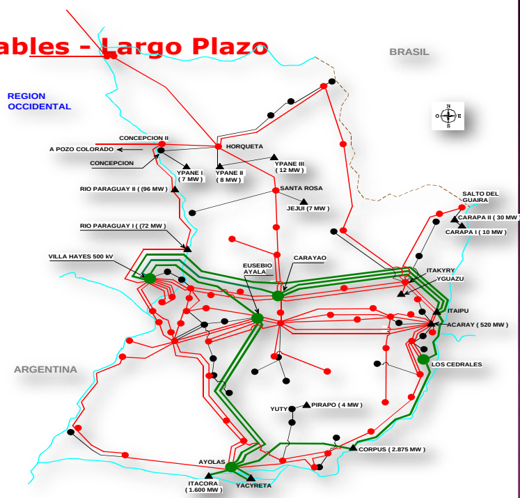
Cuadro 15 - Plano esquemático indicativo de ubicación de Futuras PCHs – Pequeñas Centrales Hidroeléctricas
