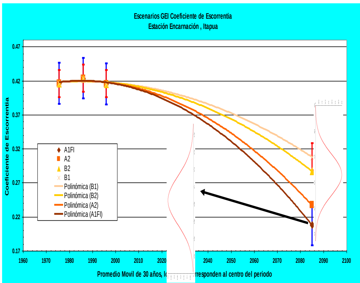
Cuadro 21 – Variación Coeficiente de Escorrentía – Período 1960 – 2085
