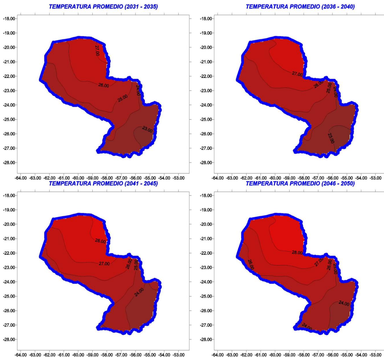
Cuadro 18 - Temperaturas promedios, estimadas para períodos consecutivos de 5 años.
